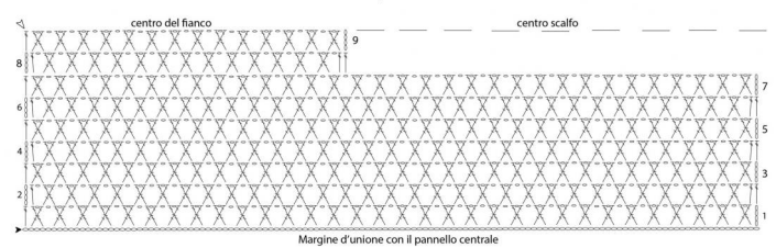
Schema 2: pannello laterale
